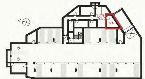
Übersicht Grundriss E-01
