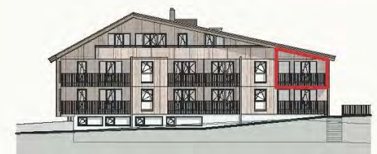
Übersicht Ansicht West
