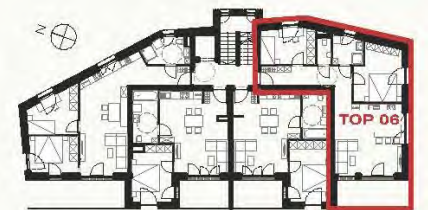
Übersicht Grundriss E01
